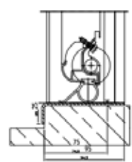
L-Bodenprofil in Edelstahl
