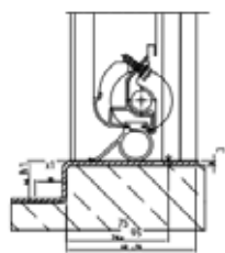
Z-Bodenprofil in Edelstahl
